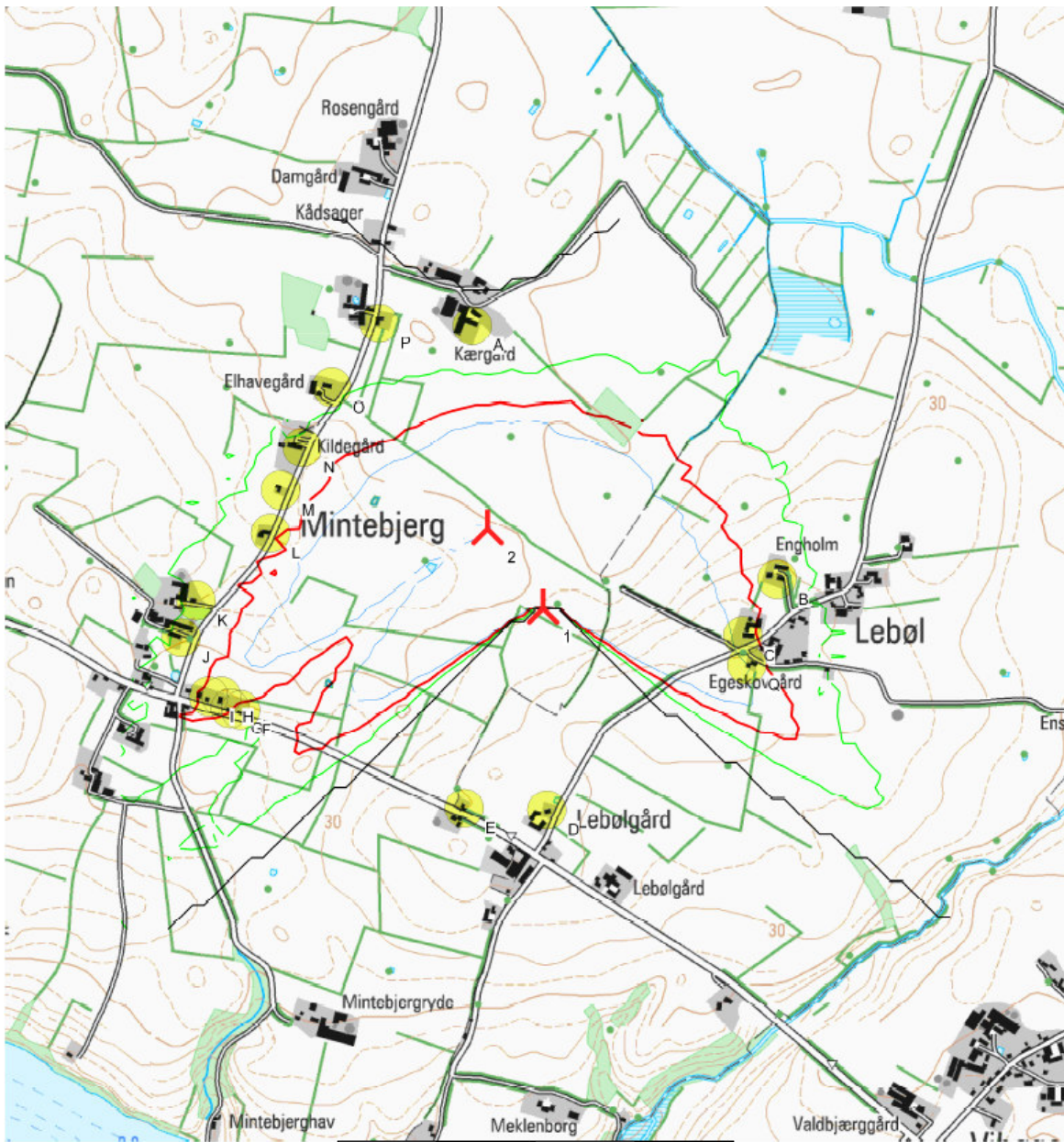
Kort: Kort25-0505_6100_560 6100_560, Udskriftsmålestok 1:15.000, Kortcentrum ETRS 89 Område: 32 Øst: 561.000 Nord: 6.084.990 ▲ Ny mølle ● Skyggemodtager Isolinier viser skygge i Timer per år, reelt tilfælde ■ 0 ■ 5 ■ 10 ■ 15
